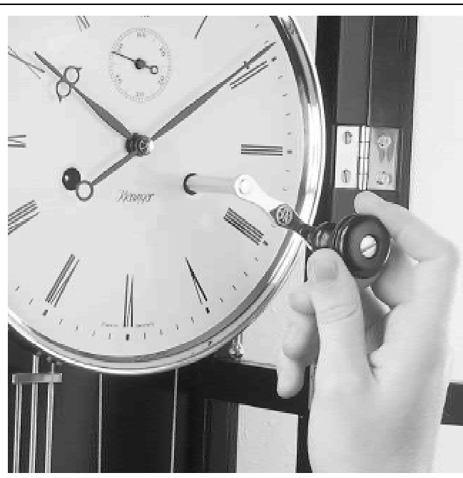
Bild 12 / Picture 12 / Figure 12 / Ilustración 12 Die Uhr aufziehen (Seilzugwerke) Winding the clock (cable movements) Remonter l'horloge (mouvements à câbles) Dar cuerda al reloj (movimiento a cable)
